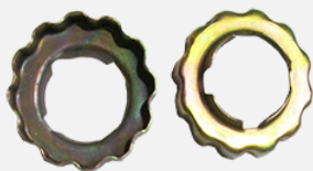
پولک خورشیدی پلوس پژو
