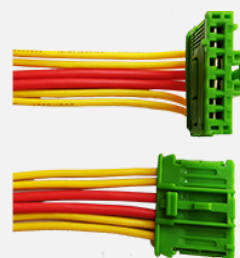
سوکت مقاومت فن 6فیش ساینا
