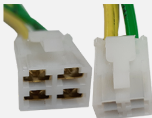
سوکت رله فن پراید انژکتور نر و ماده
